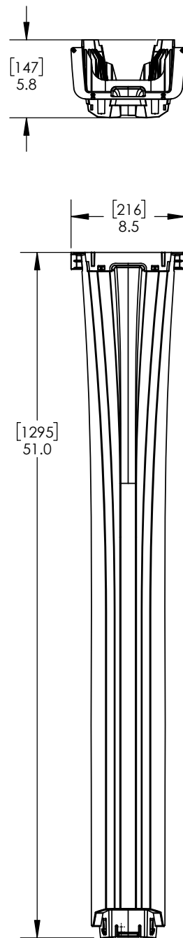
UPRIGHT OPDU52
