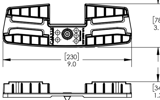
BOTTOM PLATE OPZPB
